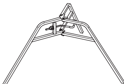
Tripod PEP Ergo, galv.
